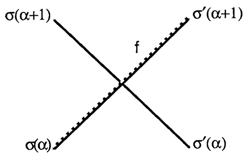
A zero singular edge for f
