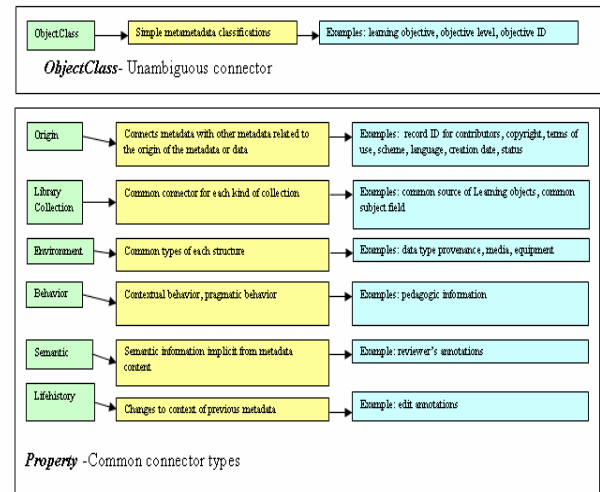
Fig. 2 Metametadata Element Concept (MeMeC)
